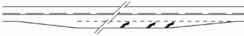
Marcajul benzii suplimentare pentru vehicule lente
